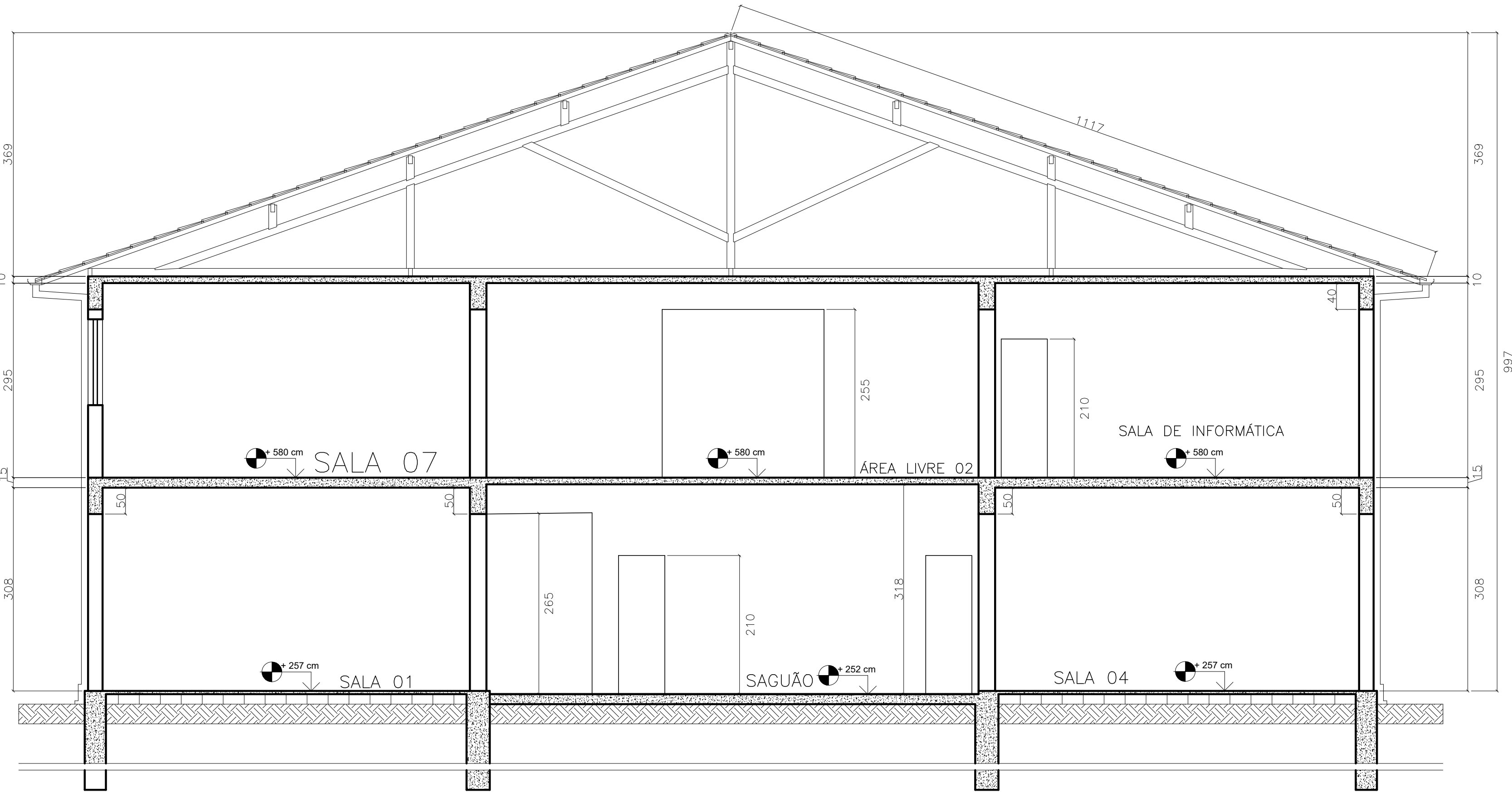
CORTE TRANSVERSAL - AB - ESCALA 1:50 MEDIDAS EM CENTÍMETROS
